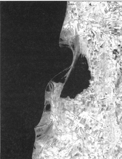
Landsat TM 1989
