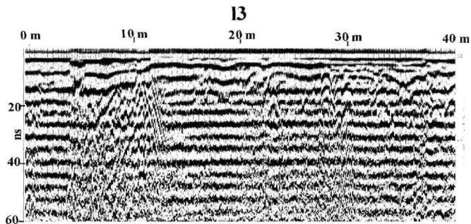
Σχ.2. Τομή κατά μήκος της οδού I3. Τα έντονα φαινόμενα περίθλασης που φαίνονται σε διάφορα τμήματα της τομής αποδίδονται στην παρουσία ανομοιογενειών στο υπέδαφος στις συγκεκριμένες θέσεις.
