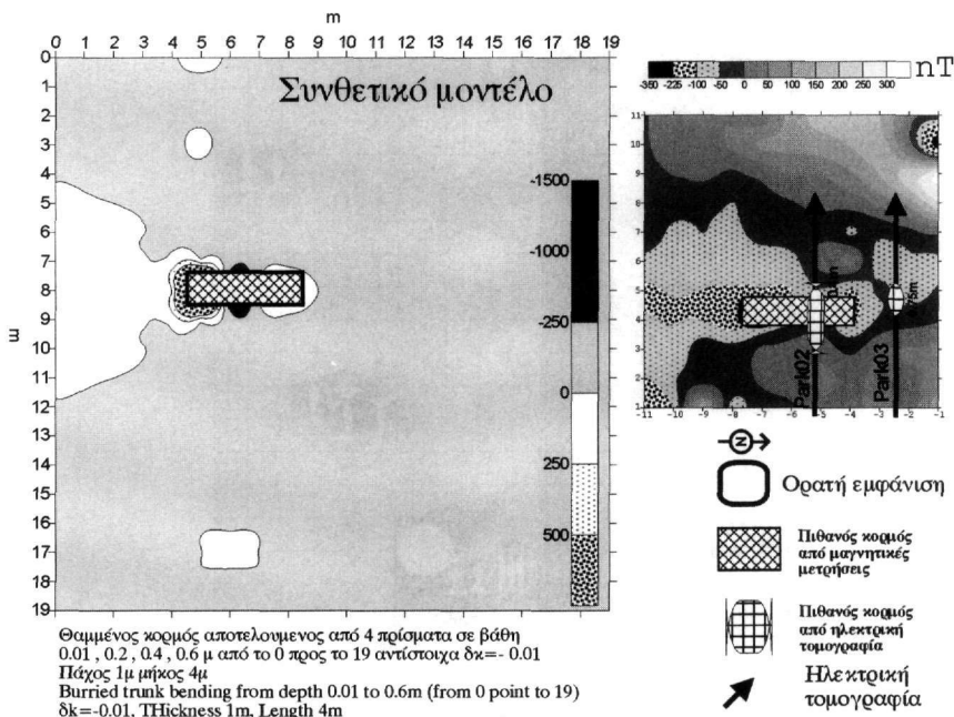
Σχ.2 Μαγνητικός χάρτης καννάβου περιοχής πάρκων απολιθωμένου δάσους. Στο αριστερό μέρος παρουσιάζεται το συνθετικό μοντέλο που κατασκευάστηκε με στόχο τη συσχέτιση με τις πραγματικές μαγνητικές μετρήσεις και τα αποτελέσματα της ηλεκτρικής τομογραφίας που παρουσιάζονται στο δεξί μέρος.
