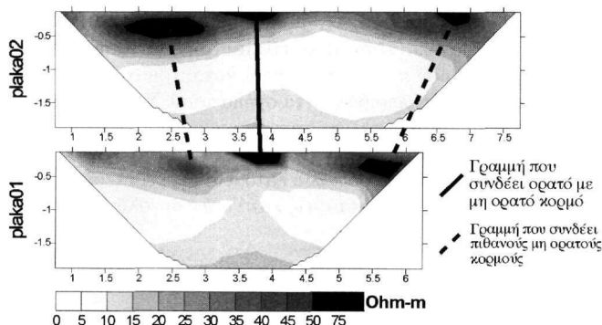
Σχ.3 Εικόνες αντιστροφής των τομογραφικών οδεύσεων plaka01 και plaka02 . Με συνεχή γραμμή συνδέεται ορατός κορμός (τομογραφία plaka01 ) με πιθανή συνέχεια του και με διακεκομμένη γραμμή συνδέονται πιθανοί μη ορατοί στόχοι που διακρίνονται στις δύο παράλληλες τομογραφίες.
