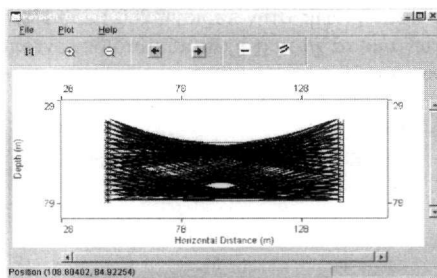
Εικόνα 5.β Κατανομή σεισμικών ακτίνων μετά την παρεμβολή σώματος κυκλικής διατομής και ταχύτητας 1000 m/s, για το ζεύγος γεωτρήσεων B1-Γ/B1-3.
