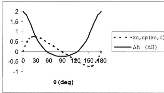
Σχ. 6. Μεταβολή των ποσοτήτων x_{0,up} , x_{0,d} , \Delta h=h'-h , \Delta H=H'-H , ως προς τη γωνία σχιστότητας, με \lambda=2 . Για τον υπολογισμό των απεικονιζόμενων μεγεθών, θεωρήθηκε ότι h=1 και H=1 .
