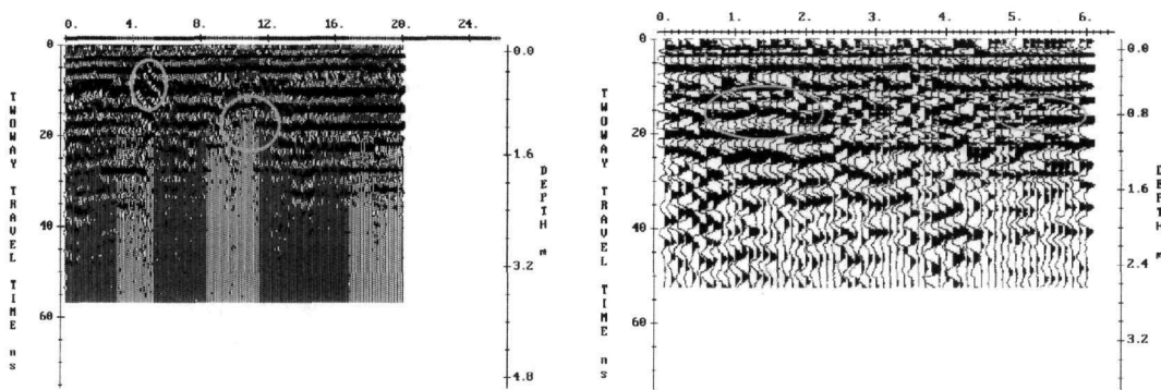
Σχ.5. Τομές γεωραντάρ στο πάρκο Μουσείου (αριστερά) και ΙΠλάκας (δεξιά) Fig. 5. GPR measurements at the park of Sigri Museum.
