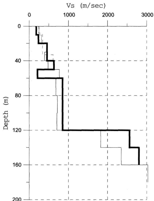
Σχήμα 8: Σύγκριση των αποτελεσμάτων της μεθόδου του μικροθορύβου (παχιά γραμμή) με τη μέθοδο SWI (απλή γραμμή) και D-H (στιγτική γραμμή)
