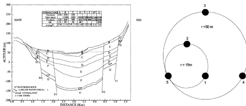
Σχήµα 1. Εδαφική τοµή Euroseistest και διάταξη καταγραφής του µικροθορύβου Figure 1. Soil profile of Euroseistest and array of the tremor recordings
