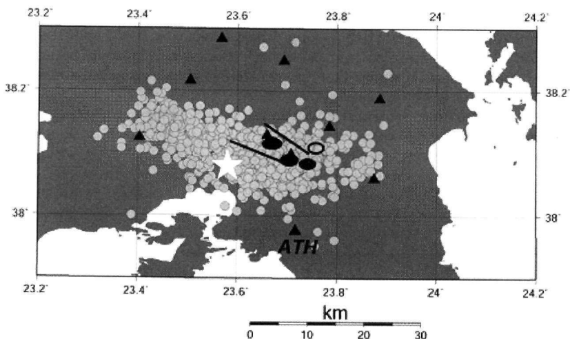
Σχήμα 1. Επίκεντρο του κύριου σεισμού (αστέρι) και επίκεντρα των μετασεισμών του πρώτου τριμήνου (κύκλοι) (δεδομένα από Papadopoulos et al., 2000). Η νότια και η βόρεια γραμμή παριστούν απλοποιημένα τα ρήγματα του Θριάσιου Πεδίου και της Φυλής, αντίστοιχα. Πρόσθετη επεξήγηση: μαύρες ελλείψεις = περιοχές μέγιστων βλαβών (Φυλή, Α. Λιόσια, Μενίδι από ΒΔ προς ΝΑ), λευκή έλλειψη = περιοχή σημαντικών βλαβών (Θρακομακεδόνες), τρίγωνα = σταθμοί αναλογικού δικτύου του Γεωδυναμικού Ινστιτούτου.
