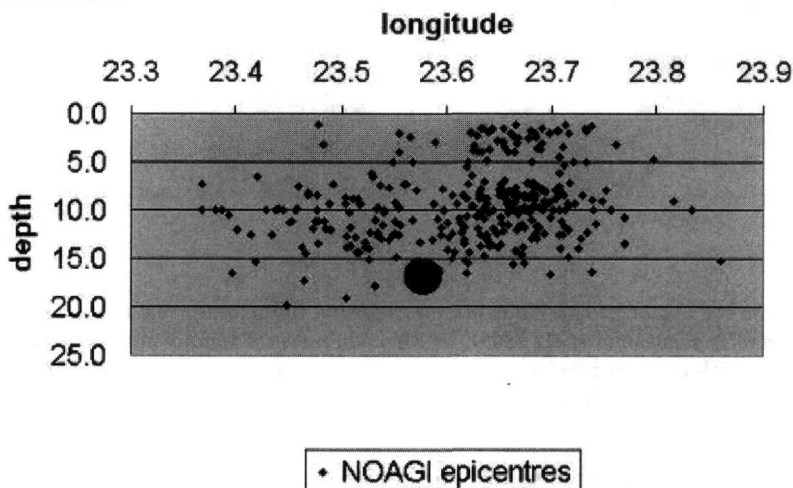
Σχήμα 2. Κατακόρυφη τομή του μετασεισμικού χώρου διεύθυνσης Α-Α. Προβάλλονται οι εστίες του κύριου σεισμού (μεγάλος κύκλος) και των μετασεισμών του πρώτου δεκαημέρου, όπως προσδιορίστηκαν από τους Papadopoulos et al. (2000, 2001).
