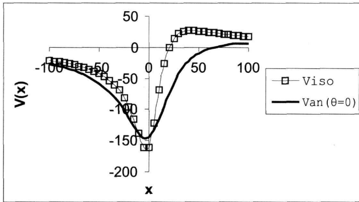
Σχ. 3. Ανωμαλία φυσικού δυναμικού για ισότροπο υπέδαφος ( V_{iso} ) και για υπέδαφος με κατακόρυφο άξονα ανισοτροπίας ( V_{an} ). Οι παράμετροι του κεκλιμένου φύλλου είναι M=100\text{mV} , h=10\text{m} , H=20\text{m} , \varphi=45^\circ . Fig. 3. Self-potential anomaly at an isotropic ( V_{iso} ) and at an anisotropic ground with a vertical anisotropy axis ( V_{an} ). M=100\text{mV} , h=10\text{m} , H=20\text{m} , \varphi=45^\circ .
