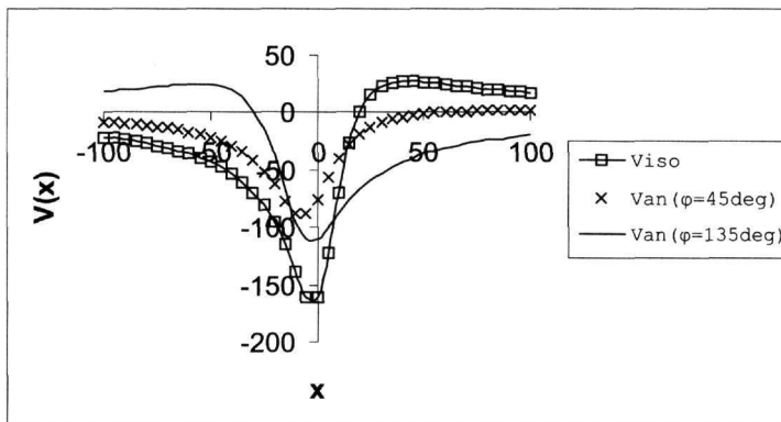
Σχ. 5. Ανωμαλίες φυσικού δυναμικού για ισότροπο και ανισότροπο υπέδαφος. Η καμπύλη V_{iso} , αντιστοιχεί σε φλέβα κλίσης \varphi=45^\circ , σε ισότροπο μέσο. Η V_{an}(\varphi=45\text{deg}) , αντιστοιχεί στην ίδια γωνία κλίσης και σε ανισοτροπία με σχιστότητα \theta=135^\circ . Η V_{an}(\varphi=135\text{deg}) , αντιστοιχεί σε γωνία κλίσης 135^\circ και σε γωνία σχιστότητας 135^\circ . Οι υπόλοιπες παράμετροι του συστήματος είναι M=100\text{mV} , h=10\text{m} , H=20\text{m} , \lambda=2 . Fig.5. Sp anomalies for an isotropic and an anisotropic ground. Curve V_{iso} , is produced by a dyke with dip angle \varphi=45^\circ , in an isotropic medium. Curve V_{an}(\varphi=45\text{deg}) , corresponds to the same dip angle, for an anisotropic ground with \theta=135^\circ . Curve V_{an}(\varphi=135\text{deg}) , corresponds to 135^\circ dip angle and to the same \theta . The system has constant parameters M=100\text{mV} , h=10\text{m} , H=20\text{m} , \lambda=2 .
