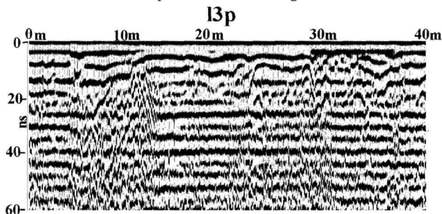
Σχ.3. Επεξεργασμένη τομή κατά μήκος της οδού I3.
