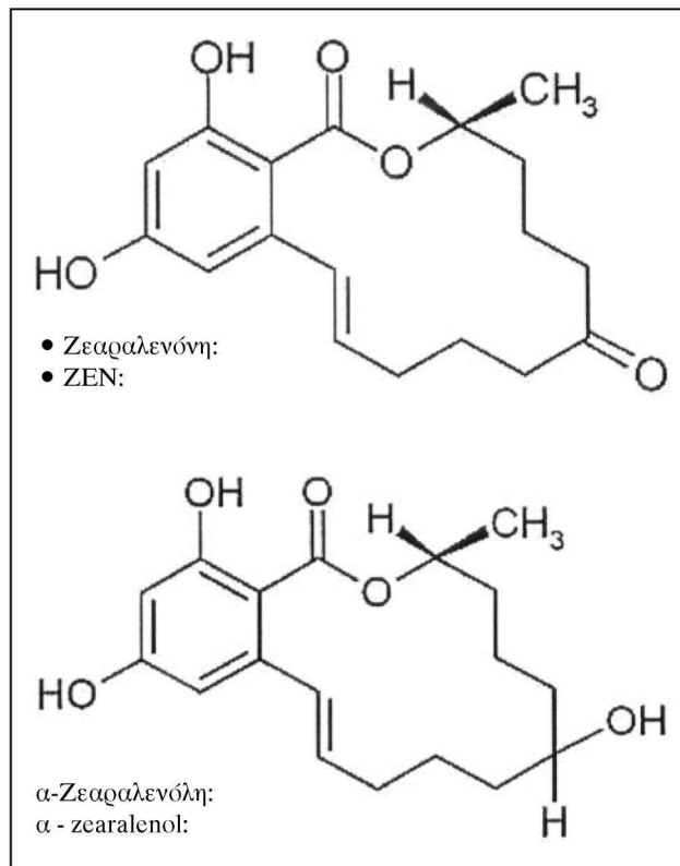
Εικόνα 3. Χημική δομή της ZEN και της α-ζεαραλενόλης (EMAN 2005δ).
