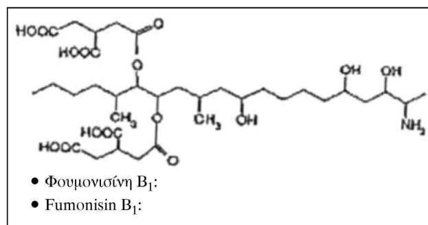
Εικόνα 5. Χημική δομή της φουμονισίνης B1 (EMAN 2005β).
