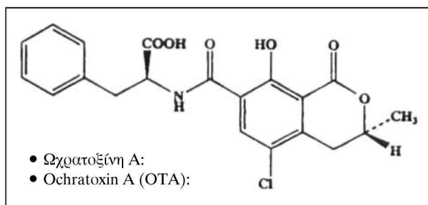
Εικόνα 4. Χημική δομή της OTA (EMAN 2005α).
