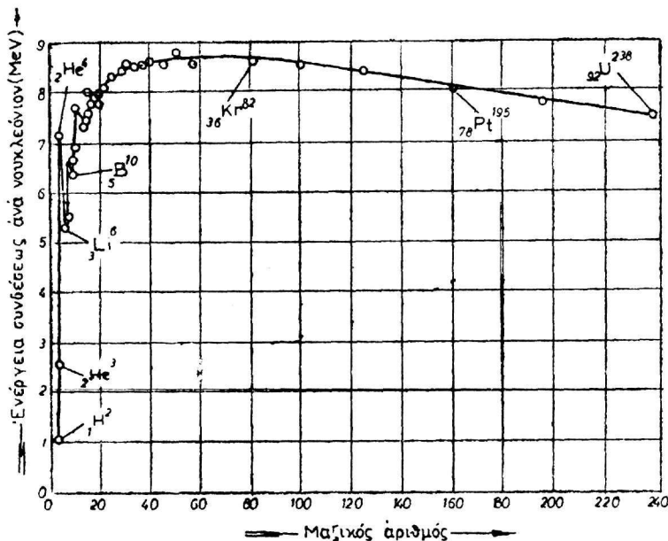
Σχ. 5.—Γραφική παράστασις ἐμφαίνουσα την ἐνέργειαν συνδέσεως ανά νουκλεόνιον των διαφόρων χημικων στοιχείων. Η ἐνέργεια συνδέσεως του Ουρανίου - 235 είναι μικροτέρα της ἐνεργείας συνδέσεως των νουκλεονίων των προϊόντων σχάσεως. Οὕτω κατά την σχάσιν ἀποδίδεται ή διαφορὰ των ἐνεργειων συνδέσεως μεταξύ προϊόντων και αντιδρώντων της αντιδράσεως.
