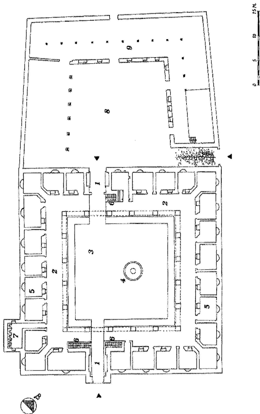
Εικ. 5. Κάτοψη του Kurşunlu Hami των Σκοπίων (Usküb). Ανασχεδίαση από Τ. Ζlatev: 1) είσοδος, 2) στοά, 3) αυλή, 4) στέρονα, 5) κελιά και εργαστήρια, 6) σκάλες ανόδου στον όροφο, 7) αποχωρητήριο, 8) εξωτερική αυλή, 9) εξωτερικοί στύλοι.
