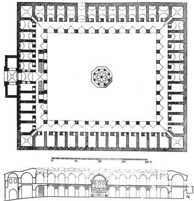
Εικ. 11. Κάτοψη και τομή του Koza Hanı της Προύσας (M. Cezar).
