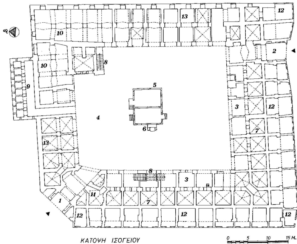
Εικ. 6. α) Κάτοψη του ισογείου του Kurşum Hanı της Φιλιππούπολης. Ανασχεδίαση από T. Zlatev: 1) κύρια είσοδος (ΒΔ), 2) δευτερεύουσα είσοδος (Ν), 3) στοά ισογείου, 4) αυλή, 5) κιόσκι, 6) κρήνη, 7) δωμάτια ισογείου, 8) σκάλα ανόδου στον όροφο, 9) χώρος αποχωρητηρίων(;), 10) επιμήκης θολοσκεπαστος χώρος, 11) δωμάτιο φύλακα ή θυρωρού, 12) μαγαζιά Δ. και Ν. πλευράς, 13) χώροι άγνωστης χρήσης (εργαστήρια;), β) Κάτοψη του ορόφου του Kurşum Hanı. Ανασχεδίαση από T. Zlatev: 1) σκάλα ανόδου στον όροφο, 2) στοά ορόφου, 3) κελιά, 4) μεγαλύτερα κελιά ή δωμάτια, 5) χώροι άγνωστης χρήσης (αποχωρητήρια;), 6) εξώστης.
