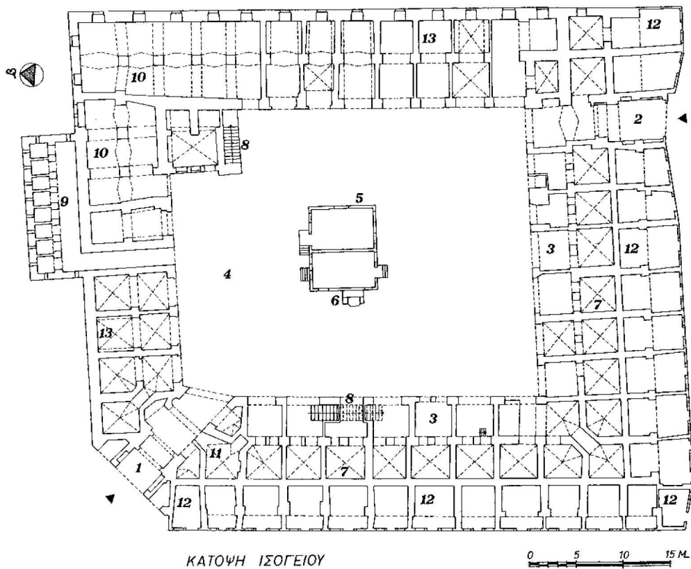
Εικ. 6. α) Κάτοψη του ισογείου του Kurşum Hanı της Φιλιππούπολης. Ανασχεδίαση από T. Zlatev: 1) κύρια είσοδος (ΒΔ), 2) δευτερεύουσα είσοδος (Ν), 3) στοά ισογείου, 4) αυλή, 5) κίοσκι, 6) κρήνη, 7) δωμάτια ισογείου, 8) σκάλα ανόδου στον όροφο, 9) χώρος αποχωρητηρίων(;), 10) επιμήκης θολοσκεπαστος χώρος, 11) δωμάτιο φύλακα ή θυρωρού, 12) μαγαζιά Δ. και Ν. πλευράς, 13) χώροι άγνωστης χρήσης (εργαστήρια); β) Κάτοψη του ορόφου του Kurşum Hanı. Ανασχεδίαση από T. Zlatev: 1) σκάλα ανόδου στον όροφο, 2) στοά ορόφου, 3) κελιά, 4) μεγαλύτερα κελιά ή δωμάτια, 5) χώροι άγνωστης χρήσης (αποχωρητήρια;), 6) εξώστης.
