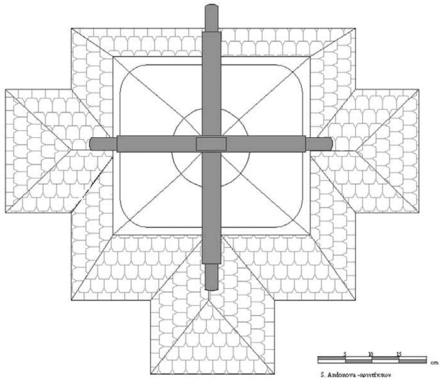
Σχ. 3. Ξύλινο πρόπλασμα κτηρίον (1795). Σχέδιο άνοψης. Sch. 3. Wooden model of building (1795). Scheme of up view.
