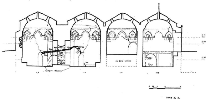
Σχ. 14α. Τομή κατά πλάτος των ζεστών χώρων ατμού.
