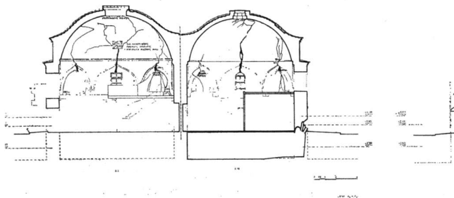
Σχ. 11. Τομή στους μεγάλους τρούλους.
