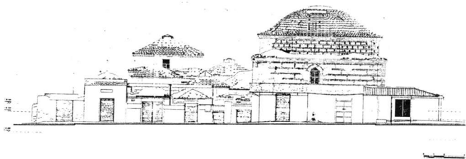
Σχ. 7. Υπάρχουσα ανατολική όψη (οδός Κομνηνών).
