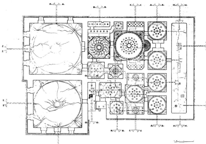
Σχ. 9. Υπάρχουσα κατάσταση των τρούλων σε άνοψη.
