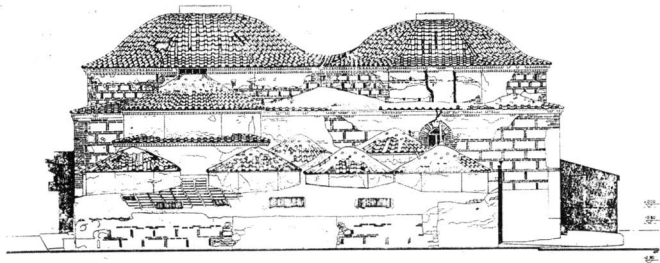
Σχ. 6. Υπάρχουσα νότια όψη (οδός Φουγκίνη).
