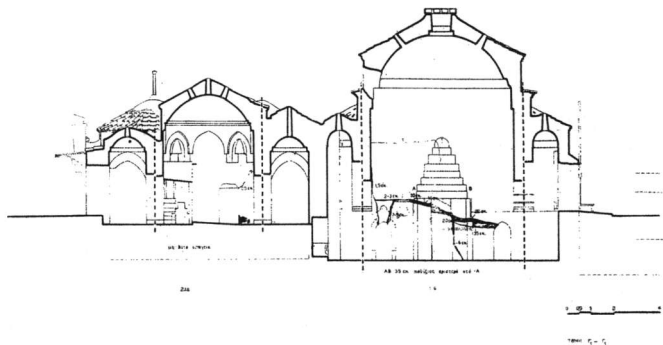
Σχ. 13. Τομή κατά πλάτος των ζεστών χώρων.
