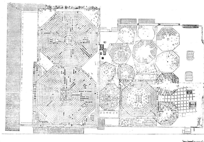
Σχ. 4. Υπάρχουσα κάτοψη τρούλων.
