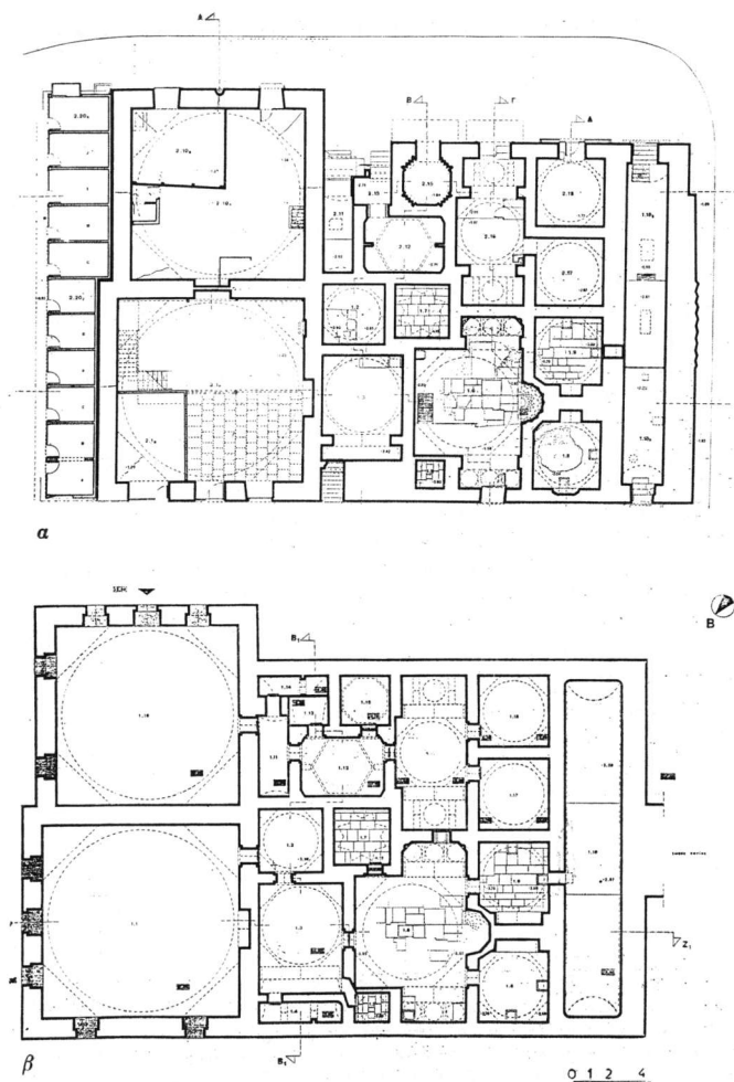
Σχ. 3. α) Υπάρχουσα κατάσταση, β) Αρχική μορφή.
