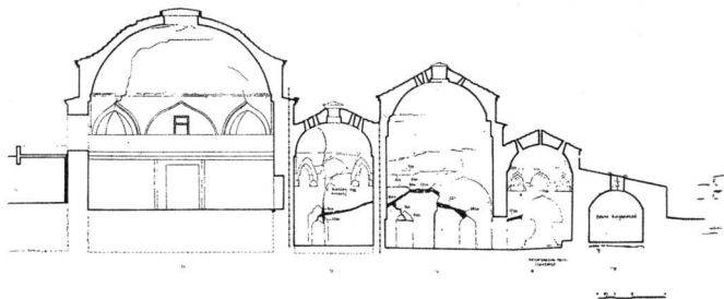
Σχ. 12. Κατά μήκος τομή.
