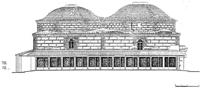
Σχ. 5. Υπάρχουσα βόρεια όψη (οδός Βασ. Ηρακλείου).
