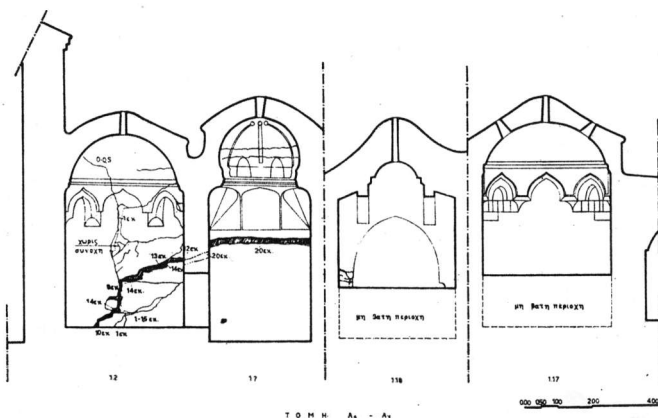
Σχ. 14β. Τομή κατά πλάτος βοηθητικών ζεστών χώρων.
