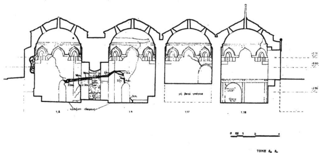
Σχ. 14α. Τομή κατά πλάτος των ζεστών χώρων ατμού.
