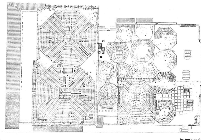
Σχ. 4. Υπόρχουσα κάτοψη τρούλων.
