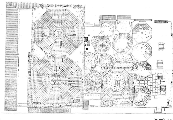
Σχ. 4. Υπόχουσα κάτοψη τρούλων.
