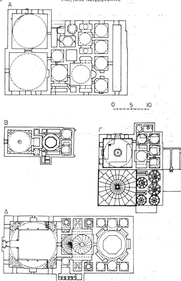
Σχ. 10. Α. Pazar ή Yahudi hamami στη Θεσσαλονίκη. Β. Cagir hamami στην Προύσα. Γ. Mustafa Paşa hamami στο Izmid. Δ. Mahmud Paşa hamami στην Κωνσταντινούπολη.
