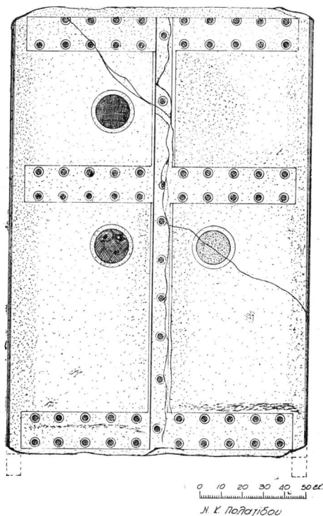
Σχέδ. 3. Πρόσωση της μαρμαρίνης θύρας
