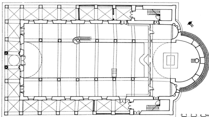
Εικ. 14. Άγιος Μηνάς Θεσσαλονίκης (1851-52). Κάτοψη. Σχέδιο Β. Κονιόρδος, 1979. Ανασχεδίαση Θ. Μαντοπούλου-Παναγιωτοπούλου, 1994.
