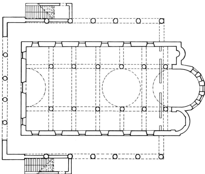
Εικ. 12. Άγιος Νικόλαος Τρανός. Κάτοψη ισογείου. Γραφική αποκατάσταση (σκαρίφημα Θ. Μαντοπούλου-Παναγιωτοπούλου).
