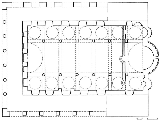
Εικ. 20. Άγιος Νικόλαος Πορταριάς Πηλίου (1855). Κάτοψη. Σχέδιο Μ. Πολυβίου.
