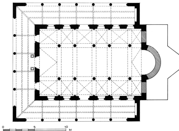
Εικ. 16. Κοίμηση Θεοτόκου Ερμούπολης (1828-1829). Κάτοψη ισογείου. Γραφική αποκατάσταση του αρχικού σχεδίου. Πηγή: Ι. Τρανού - Α. Κόκκου, Ερμούπολη, Αθήνα 1980, σ. 89.
