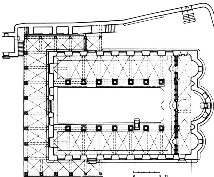
Εικ. 18. Παναγία Αγιάσου Μυτιλήνης (1815). Κάτοψη. Πηγή: Ι. Γ. Κλεομβρότου, Mytilena sacra , τ. 2, Θεσσαλονίκη 1974, πίν. Ι.
