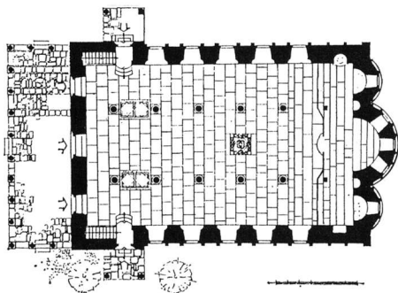
Εικ. 24. Άγιος Πέτρος και Παύλος Sorot Βουλγαρίας (1848). Κάτοψη. Πηγή: M. Koeva, Cultural Monuments of the Bulgarian National Revival Period , Sofia 1977, σ. 137.
