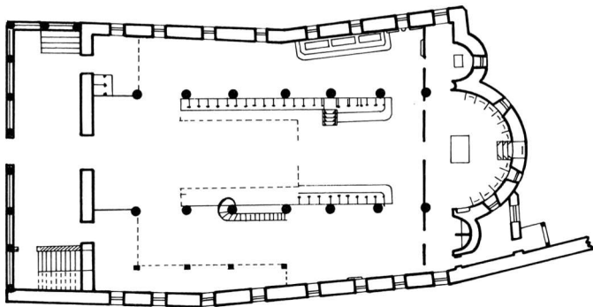
Εικ. 22. Πατριαρχικός ναός αγίου Γεωργίου Κωνσταντινούπολης (οικοδόμηση 1720 - ανακαίνιση 1836). Κάτοψη. Πηγή: Μητρ. Ελβετίας Δαμασκηνού - Β. Φειδά - Α. Πασαδαίου - Α. Παλιούρα, Το Οικουμενικό Πατριαρχείο, Αθήνα 1989, σ. 69.
