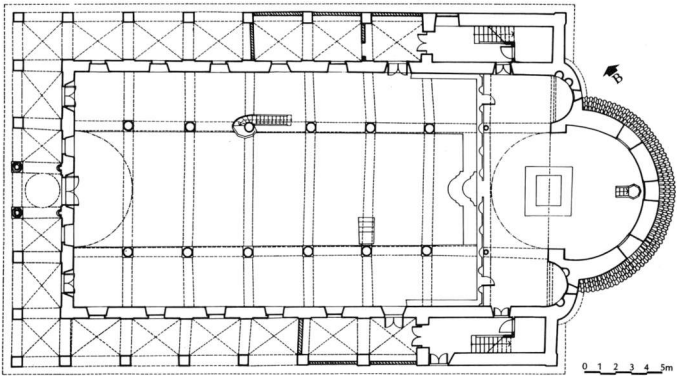
Εικ. 14. Άγιος Μηνάς Θεσσαλονίκης (1851-52). Κάτοψη. Σχέδιο Β. Κονιόρδος, 1979. Αναθεώρηση Θ. Μαντοπούλου-Παναγιωτοπούλου, 1994.
