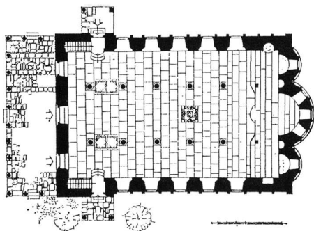
Εικ. 24. Άγιος Πέτρος και Παύλος Σοροτ Βουλγαρίας (1848). Κάτοψη. Πηγή: M. Koeva, Cultural Monuments of the Bulgarian National Revival Period , Sofia 1977, σ. 137.
