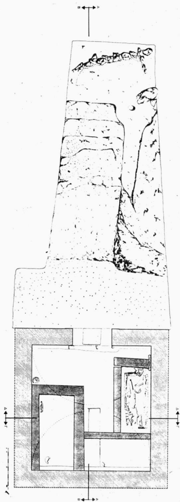
Σχέδ. 1. Η κάτοψη του τάφου και η λαξευμένη κλίμακα.
