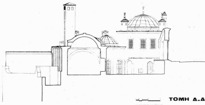
Σχ. 8. Τομὴ Δ-Δ. Κατὰ πλάτος τομὴ στὸ Ἱμαρέτ-μεκτέμπ
