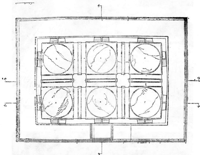
Σχ. 1. Κάτοψη του Μπεζεστενίου Θεσσαλονίκης (σχ. αρχιτ. Ε. Χ'τρίφορος, Ε. Κατσανίκα, Κ. Θεολογίδου).
