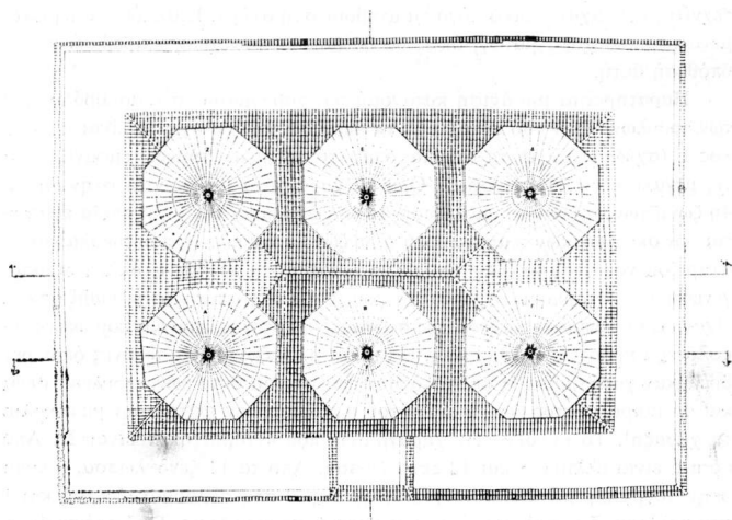
Σχ. 2. 'Ανοψη στέγης του Μπεζεστενίου Θεσσαλονίκης. Διακρίνονται οι 4 ζώνες των φύλλων μολυβιού (σχ. άρχιτ. Ε. Χ' τρύφωνος, Ε. Κατσανίνα, Κ. Θεολογίδου).
