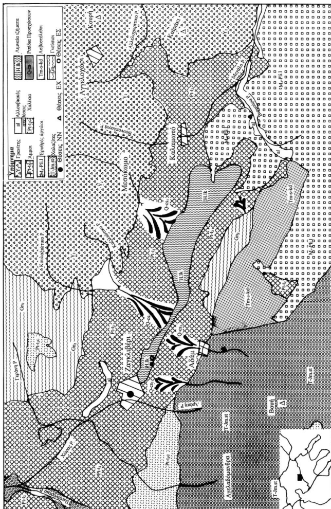
Σχ. 1. Γεωλογικός χάρτης περιοχής Ζαγκλιβεριού.
