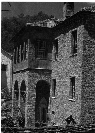
Εικ. 26. Αγία Σωτήρα Βοΐου: πέτρι- να τόξα (φωτ. του συγγρα- φέα, 1991).
