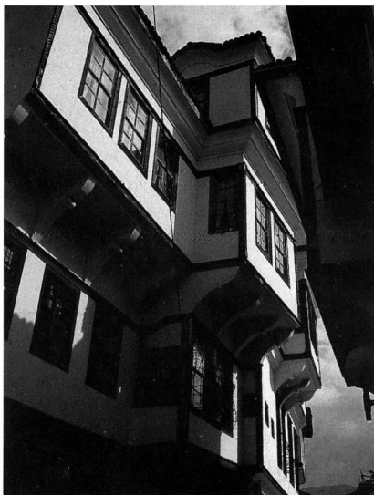
Εικ. 17. Αχρίδα: άποψη του αρχοντι- κού Ρόμπη. Διακρίνονται τα επάλληλα σαχνισιά της βόρειας πτέρυ- γας του κτιρίου (φωτ. του συγγρα- φέα, 1999).
