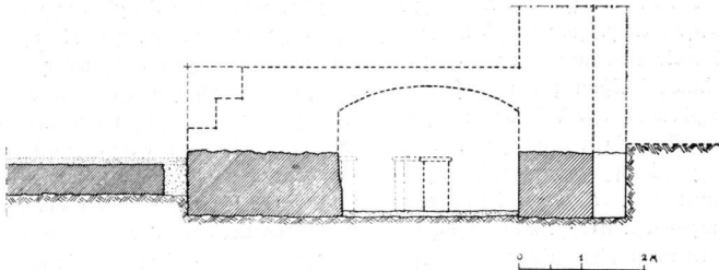
Σχ. 3. Κατακόρυφη τομή του υπόγειου διαδρόμου του Ιερού σε υποθετική αναπαράσταση.
