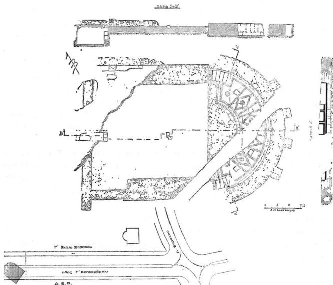
Σχ. 2. Κάτοψη του Ιερού Βήματος του ναού.
