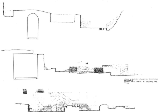
Σχ. 9. Ἡ Τομή τοῦ λουτροῦ τῆς οδοῦ Μαβίλη 9.
