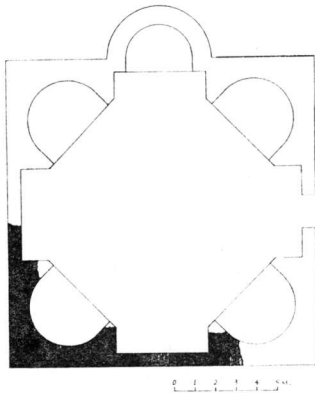
Σχ. 6. Κάτοψη τοῦ βαπτιστηρίου.
