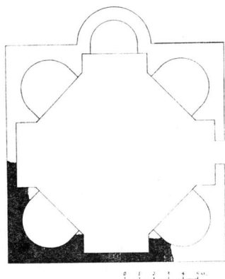
Σχ. 6. Κάτοψη του βαπτιστηρίου.
