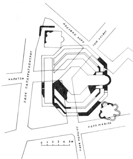
Σχ. 5. Τοπογραφικὸ τοῦ συγκροτήματος τοῦ Ὀκταγώνου μετὰ τὸ βαπτιστήριο καὶ τὸ μαρτύριο.
