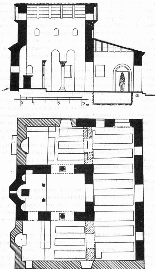
Εικ. 1. "Άγιος Νικόλαος Ὁρφανός. Κάτοψις καὶ τομὴ τοῦ ναοῦ μετὰ τὰς γενομένης ἐργασίας.
