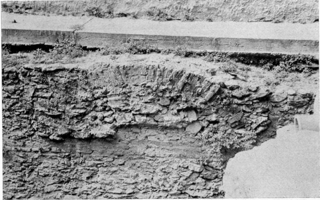
α. Τὸ ἀνακουφιστικὸ τῶξο στὸ νότιο στελοβάτη τοῦ κεντρικοῦ κλίτους τοῦ ναοῦ Α
