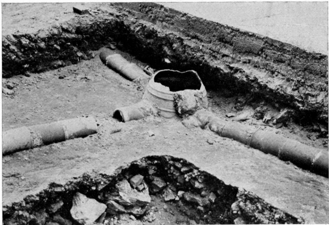
β. Τὸ ἀποχετευτικὸ σύστημα μὲ τοὺς κυλινδρικοὺς σωλήνες
