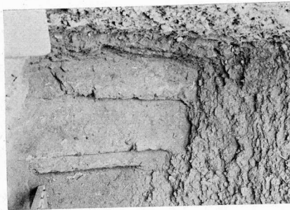
β. Ὁ τοῖχος H1 καὶ οἱ βαθμίδες μετὰ τὸ πατημένο πηλόχωμα
