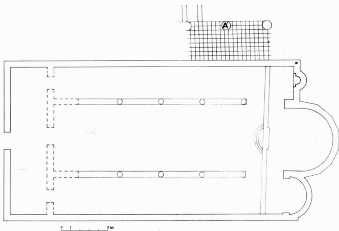
Σχ. 1. Ἡ κάτοψη τοῦ καμένου ἀπὸ τὴν πυρκαγιά τοῦ 1917 ναοῦ τοῦ Ἁγίου Νικολάου Τρανοῦ.
