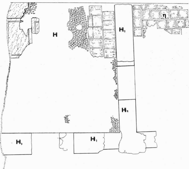
Σχ. 5. Ἡ κάτωψη τῆς ὑστερορωμαϊκῆς αἴθουσας H
