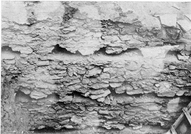
β. Ἡ τοιχοδομία τοῦ τοίχου Β1
