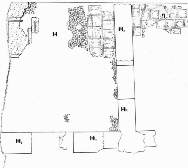
Σχ. 5. Ἡ κάτωψη τῆς ὑστερορωμαϊκῆς αἴθουσας Η
