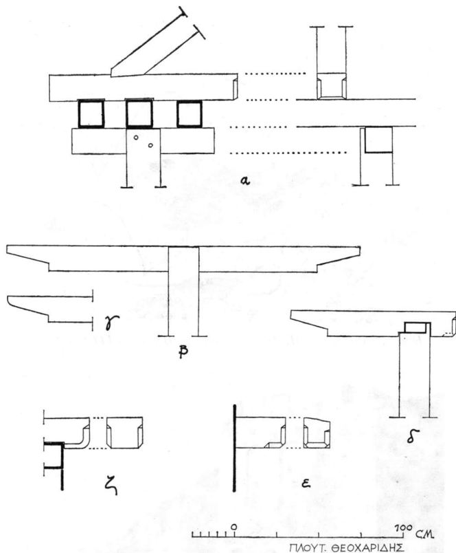
Σχ. 7. Λεπτομέρειες ξύλινων οικοδομικών στοιχείων: α. η δυτική έδραση τής στέγης του βόρειου σκέλους τής ανατολικής πτέρυγας (στύλος, κιονόκρανο, επιστύλια, τακούνι, ψαλίδι). β. τυπικό κιονόκρανο του πρόσθετου ΝΔ κτίριου (ή διάσταση του μήκους ποικίλλει, βλ. εικ. 3). γ. σπανιότερη παραλλαγή στην καταγρασία του προηγούμενου. δ. στύλος και έκκεντρο κιονόκρανο έντοιχισμένα στην έξωτερική όψη του δυτικού τοίχου, στον άνωτατο όροφο του πρόσθετου ΝΔ κτίριου (βλ. σ. 454, σημ. 1). ε. οριζόντιο γωνιακό φουρούσι στέγης, στη ΝΔ γωνία τής παλιότερης νότιας πτέρυγας. ζ. τακούνι στέγης στο νότιο άκρο του κεντρικού σκέλους τής ανατολικής πτέρυγας, πλευρά ανατολική
