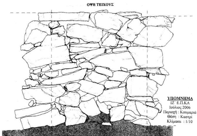
Εικ. 3. Μεγάλο Καστρί. Σχεδιαστική απόδοση εξωτερικής πλευράς τμήματος τείχους στον βόρειο λόφο.
