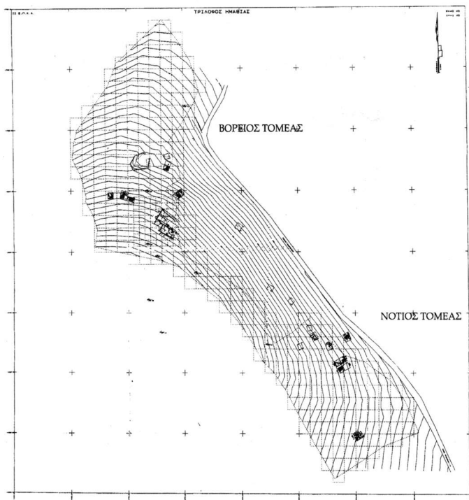
Εικ. 4. Μπας Καρτέρ. Τοπογραφική αποτύπωση της ανατολικής πλευράς του λόφου με τη θέση των δοκιμαστικών τομών (2006).
