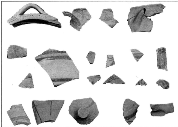
Εικ. 5. Κοζάνη, μυκηναϊκά όστρακα.
