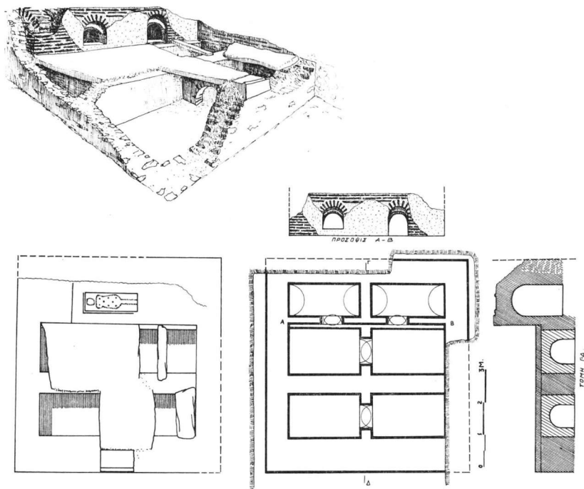
Σχέδ. 8. Ταφικό συγκρότημα του ανατολικού νεκροταφείου (57).
