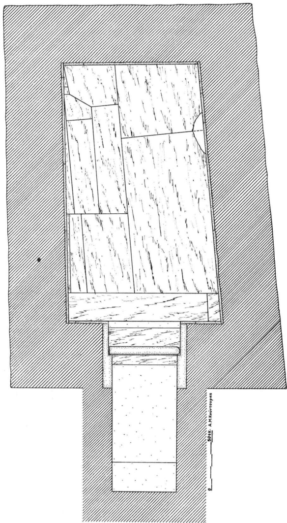
Σχ. 3. Κάτωψη χτιστού τάρου του ανατολικού νεκροταφείου (57).
