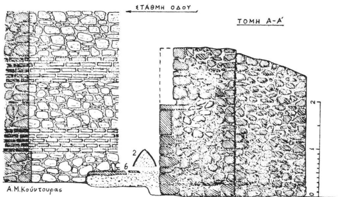
Σχέδ. 11. Τομή καὶ ὄψη τοῦ τείχους καὶ πυργοειδοῦς τριγωνικῆς ἐξοχῆς (59).
