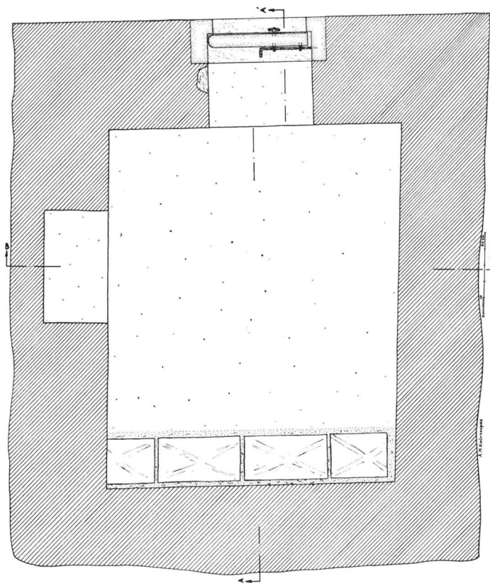
Σχέδ. 5. Κάτοψη κτιστοῦ τάφου (57).
