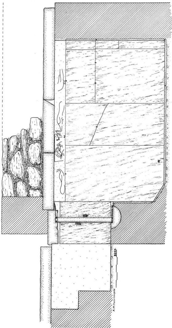
Σχέδ. 4. Τομή κατά μήκος του τάφου του σχεδ. 3 (57).
