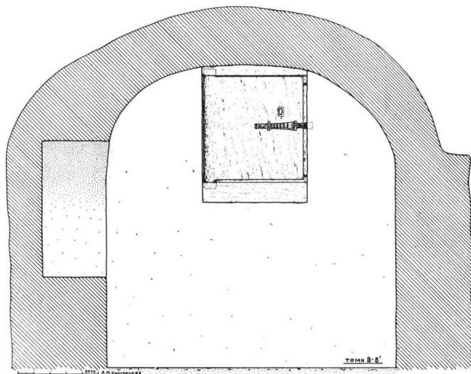
Σχέδ. 7. Τομὴ κατὰ πλάτος τοῦ τάφου τοῦ σχεδ. 5 (57).
