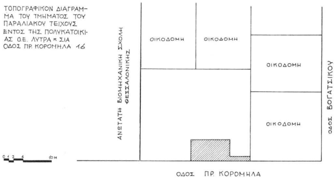
Σχέδ. 13. Τοπογραφικὸ διάγραμμα μετὰ τὰ λείψανα πύργου τοῦ παραλιακοῦ τείχους (59).
