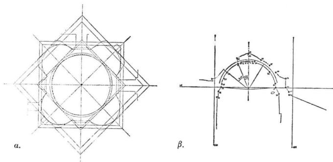
Σχ. 10. α: χάραξη κάτοψης ζεστού χώρου, β: ο τοούλος.
