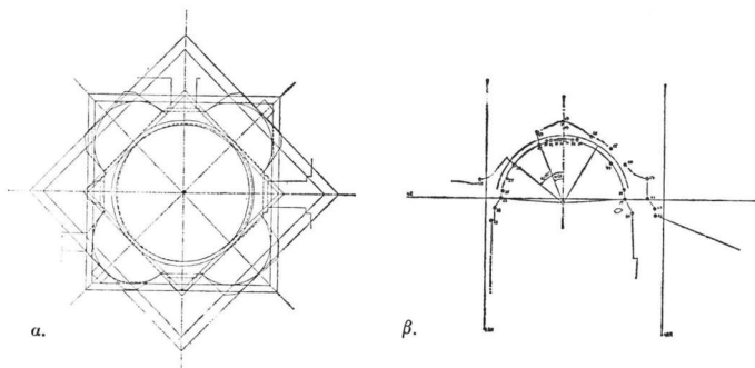
Σχ. 10. α: χάραξη κάτοψης ζεστού χώρου, β: ο τρούλος.
