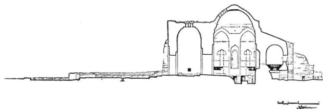
Σχ. 4. Η κατά μήκος τομή (υπάρχουσα κατάσταση).
