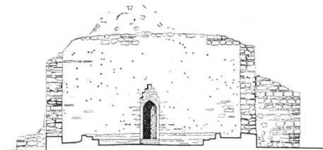
Σχ. 2. Η νότια όψη (υπάρχουσα κατάσταση).
