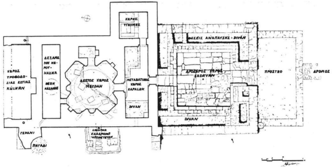
Σχ. 1. Κάτοψη: οι χώροι.
