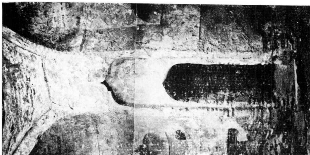
β. Η είσοδος από το ζεστό χώρο στον ατομικό χώρο (αποτίχιση). Επάνω (βέλος) φαίνεται το στόμιο (κλεισμένο) αεριογωγού.
