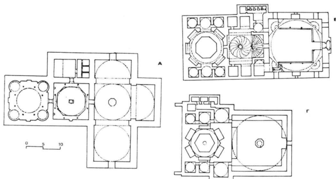
Σχ. 11. A: Eski-Karlica (Προύσα), B: Mahmut-paşa-hamami (Κων/πολη), C: Kılıçalı-paşa-hamami (Κων/πολη) (σχέδια κατά Klinghardt).
