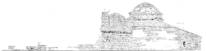
Σχ. 7. Αποκατάσταση: ανατολική όψη.
