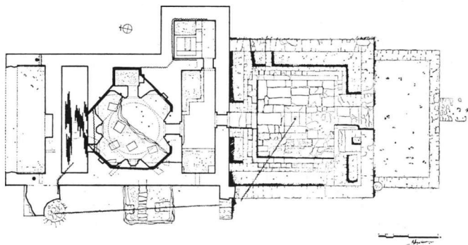
Σχ. 5. Σχέδιο λειτουργίας (ζεστό, κρύο, νερό, ζεστός αέρας) (τεθλασμένη: κρύο νερό, τελείες: ζεστό νερό).
