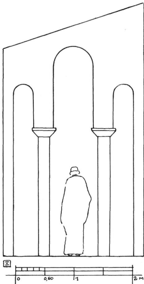
Εἰκ. 2. Ναὸς Ταξιαρχῶν. Ἀποκατάστασις τῆς ἀρχικῆς μορφῆς τοῦ τριλόβου ἀνοίγματος εἰς τὸν ἀνατολικὸν τοίχον τῆς Προθέσεως.
