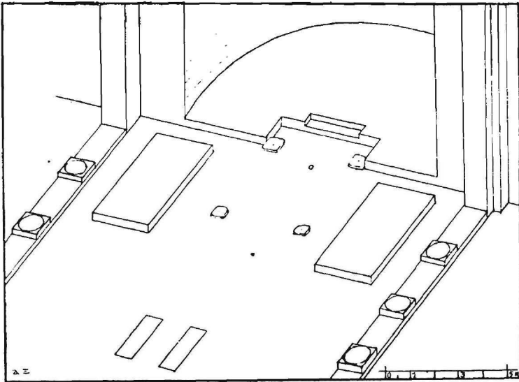
Εἰκ. 4 Ἴσομετρικὴ ἀπεικόνισις τῶν εἰς τὸ Ἱερὸν Βῆμα τῆς Ἀχειροποιήτου ἀνευρεθέντων κτισμάτων.
