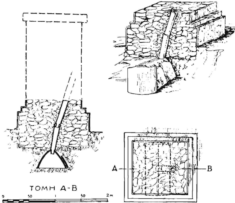
Εἰκ. 4. Βωμός ἐν Θεσσαλονίκῃ μετ' ἀγωγῶ χῶv.
