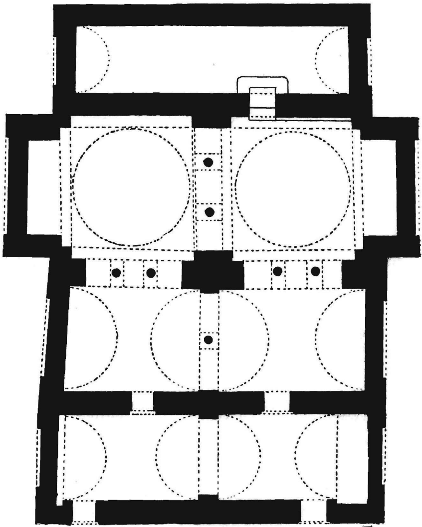
Είκ. 7. Βυζαντινός λουτρών εν Θεσσαλονίκη. Κάτοψις.
