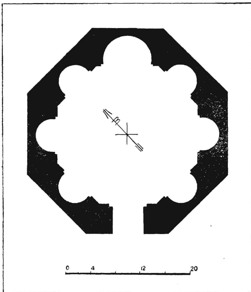
Εἰκ. 1. Κάτοψις συμπληρωμένη τοῦ ὀκταγώνου τῆς Θεσσαλονίκης.
