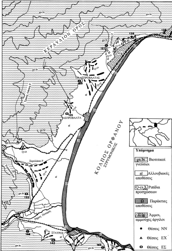
Σχ. 1. Γεωλογικός χάρτης περιοχής Ασπροβάτας.
