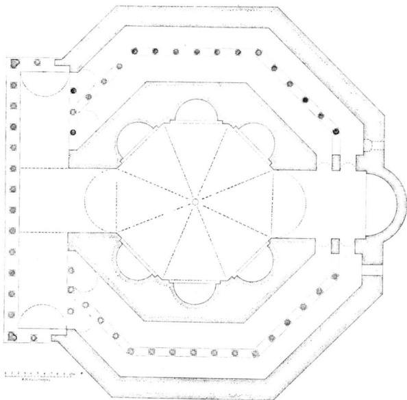
Σχ. 8. Κάτοψη του 'Οκταγώνου.
