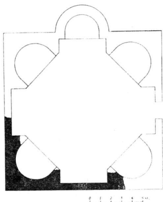
Σχ. 6. Κάτοψη τοῦ βαπτιστηρίου.
