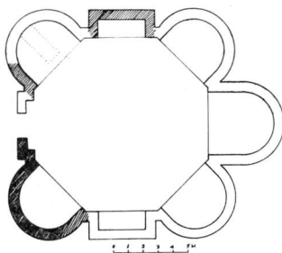
Σχ. 7. Κάτοψη τοῦ μαρτυρίου τοῦ συγκροτήματος.
