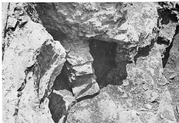
β. Ἀποψη τοῦ praefurnium τοῦ λουτροῦ τῆς ὁδοῦ Πηγειοῦ 8.
