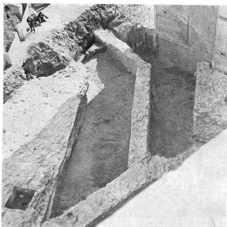
α. Ἀποψη τῶν θεμελιώσεων τοῦ ἐσωτερικοῦ πυρήνα, τοῦ στυλοβάτη καὶ τοῦ ἐξωτερικοῦ τοίχου τοῦ ὀκταγώνου στὰ θεμέλια οἰκοδομῆς τῶν ὁδῶν Κάλβου, Καρατζᾶ καὶ Πηγειοῦ. Διακρίνεται ἀριστερὰ ἡ τετράγωνη κινστέρινα καὶ δεξιὰ τὸ φρεάτιο.
