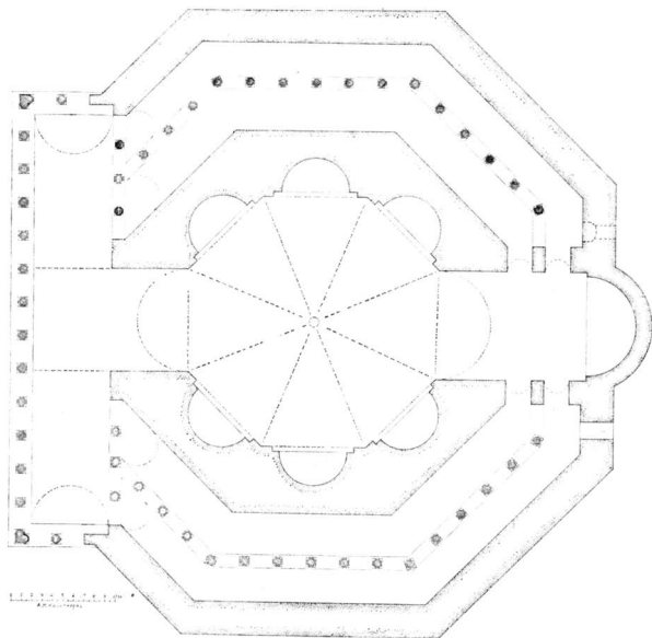
Σχ. 8. Κάτοψη τοῦ Ὀκταγώνου.
