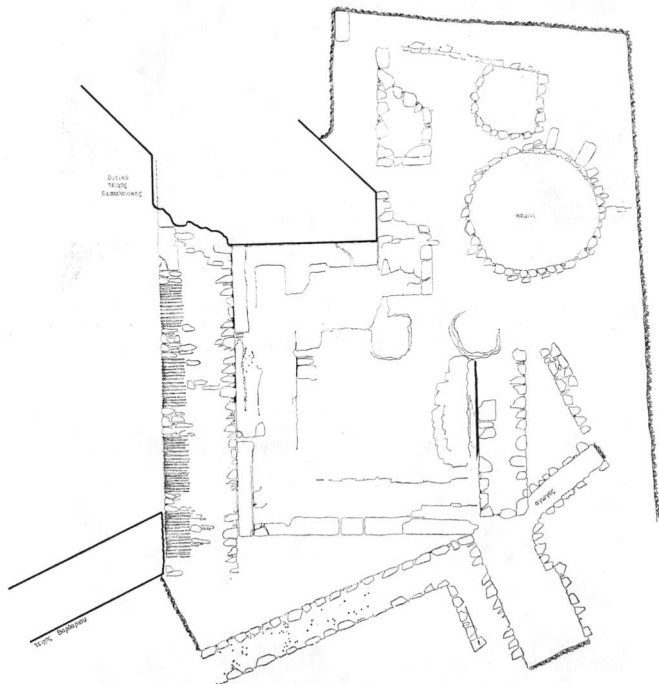
Σχ. 1. Κάτοψη ὀρθογωνίου πύργου καὶ βυζαντινοῦ κεραμικοῦ φούρνου, ποὺ ἀνασκάφηκε στὴ συμβολὴ τῶν ὁδῶν Φράγκων καὶ Μοσκόφ. Τὸ σχέδιο τοῦ πύργου ἔγινε ἀπὸ τὴν Κ. Θεοχαρίδου καὶ τοῦ κεραμικοῦ κλιβάνου ἀπὸ τὴν Ν. Ἰωαννίδου
