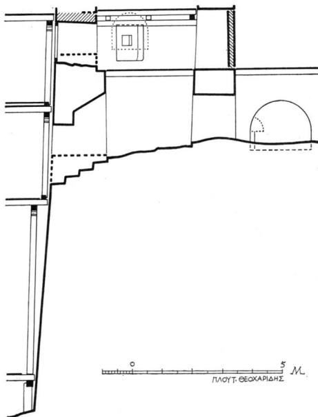
Σχ. 5. Τομή τοῦ ὀρθογωνικοῦ προμαχώνα τής παλιότερης νότιας πτέρυγας
