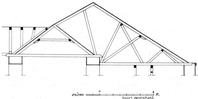
Σχ. 8. Τομή τῆς στέγης τοῦ νότιου σκέλους τῆς ἀνατολικῆς πτέρυγας καὶ τῆς μεταγενέστερης στέγης τοῦ πρόσθετου ΝΑ κτίριου
