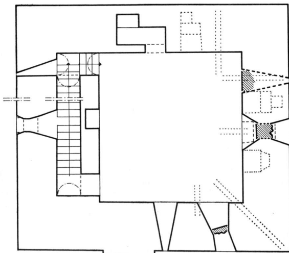
Εικ. 8. Ὁ ἀνατολικὸς τοῖχος στὸ ἐσωτερικὸ τοῦ προτελευταίου ὄροφου τοῦ πύργου (βλ. σ. 468, σημ. 1)
