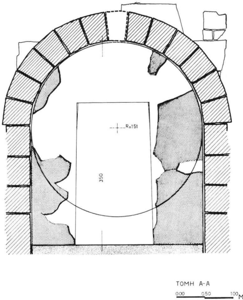
Σχέδ. 4. Ἡ τομὴ Α-Α τοῦ τάφου
