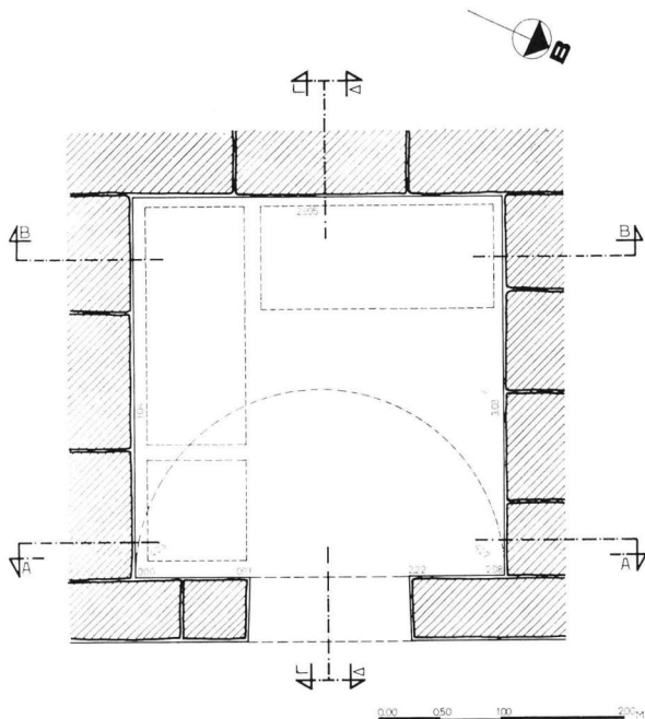
Σχέδ. 2. Κάτοψη τοῦ τάφου
