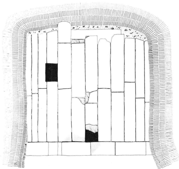
Σχέδ. 5. Όψη τής καμάρας του τάφου από πάνω
