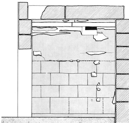
Σχέδ. 6. Ἡ τομὴ Γ-Γ' τοῦ τάφου
