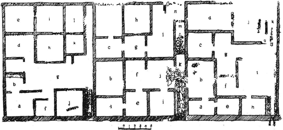
Εἰκ. 2.— Οἰκίαις A 11 - 13 (= Hel. h. πίν. 91).
