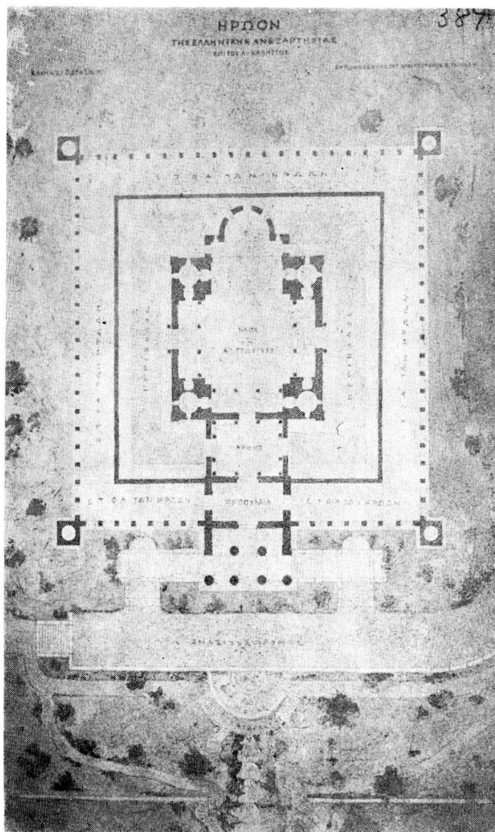
7. Ernest Ziller, 'Ηρώον τῆς Ἑλληνικῆς Ἀνεξαρτησίας ἐπὶ τοῦ Λυκαβηττοῦ, κάτοψη, φωτογ. ἀριθ. 233α, ἀπὸ το Ἀρχεῖο τῆς Εθνικῆς Πινακοθήκης
