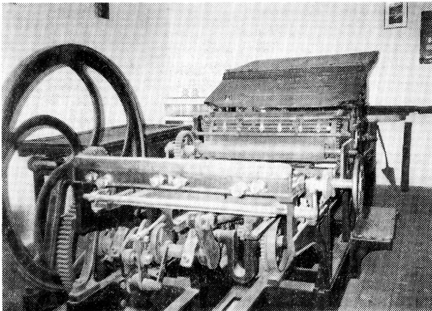
Ἐπίπεδο χειροκίνητο πιεστήριο, σχῆμα 52×82 ἐκ., Maschinenfabrik Augsburg, 1882. Λειτουργήσε στὸ Ἀγιορειτικὸ Τυπογραφεῖο ἀπὸ τὸ 1930 ἕως τὸ 1953. (Φωτογρ. Χρῆστος Μανουσαρίδης, 1996)
