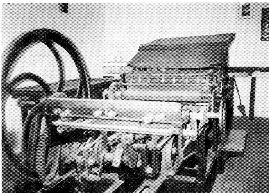
Ἐπίπεδο χειροκίνητο πιεστήριο, σχῆμα 52 × 82 ἐκ., Maschinenfabrik Augsburg, 1882. Λειτουργήσε στὸ Ἀγιορειτικὸ Τυπογραφεῖο ἀπὸ τὸ 1930 ἕως τὸ 1953. (Φωτογρ. Χρῖστος Μανουσαριδῆς, 1996)
