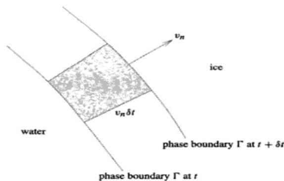
Σχήμα 1.1. Η συνθήκη Stefan
