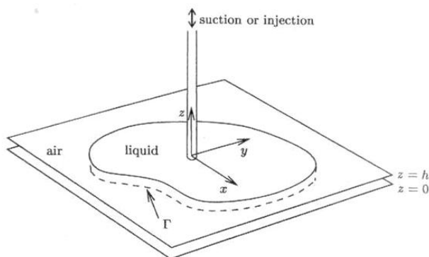
Σχήμα 1.2. Ένα κελί Hele-Shaw
