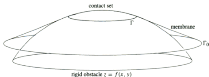
Σχήμα 1.3. Πρόβλημα εμποδίου για μία μεμβράνη
