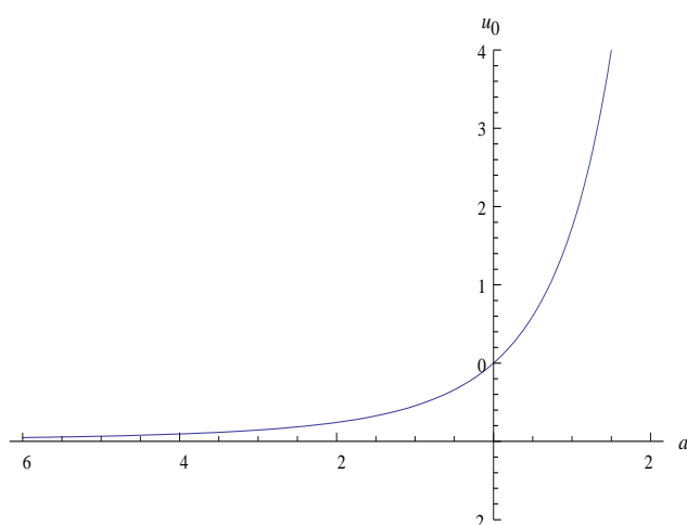
Σχήμα 3.1. Η κρίσιμη τιμή της θερμοκρασίας στο πρόβλημα Stefan
