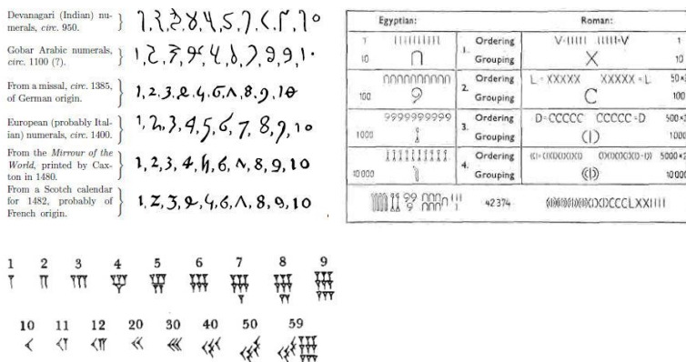
Σχήμα 3: Αριθμητικά συστήματα; (α) Ινδοαραβικό – (β) Αιγυπτιακό -Ρωμαϊκό –(γ) Βαβυλωνιακό στο Menninger (2013).
