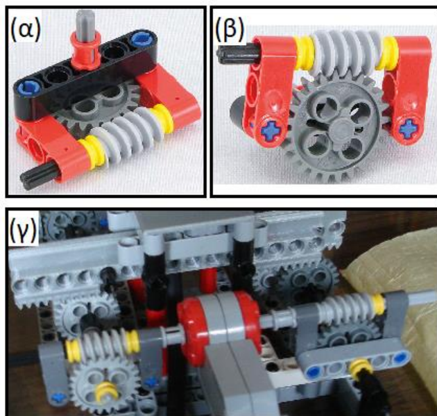
Εικόνα 6: (α και β) Συνδυασμός γραναζιών για να πετύχουμε την επιθυμητή ακρίβεια στην κίνηση της κάθε ράγας. (γ) Η κάθε ράγα στηρίζεται και στις δύο μεριές της σε γρανάτζι που περιστρέφονται από τον ίδιο κινητήρα.
