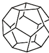
Δωδεκάεδρο
