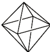
Οκτάεδρο
