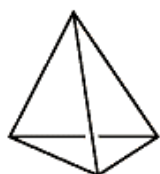
Τετράεδρο
