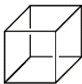
Κύβος
