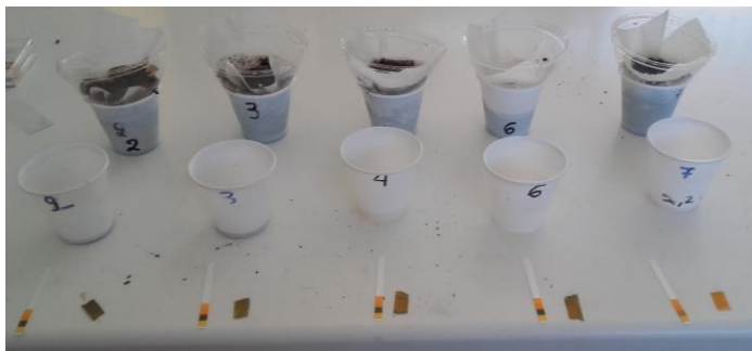
Εικόνα 4: Πειραματική διαδικασία για τον προσδιορισμό του pH σε δείγματα χώματος.
