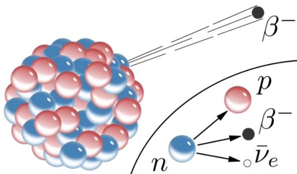
Σχήμα 5: Διάσπαση \beta^- : Νετρόνιο μετατρέπεται σε πρωτόνιο, ηλεκτρόνιο και αντινεutrίνο
