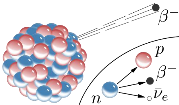
Σχήμα 5: Διάσπαση β - : Νετρόνιο μετατρέπεται σε πρωτόνιο, ηλεκτρόνιο και αντινεutrίνο
