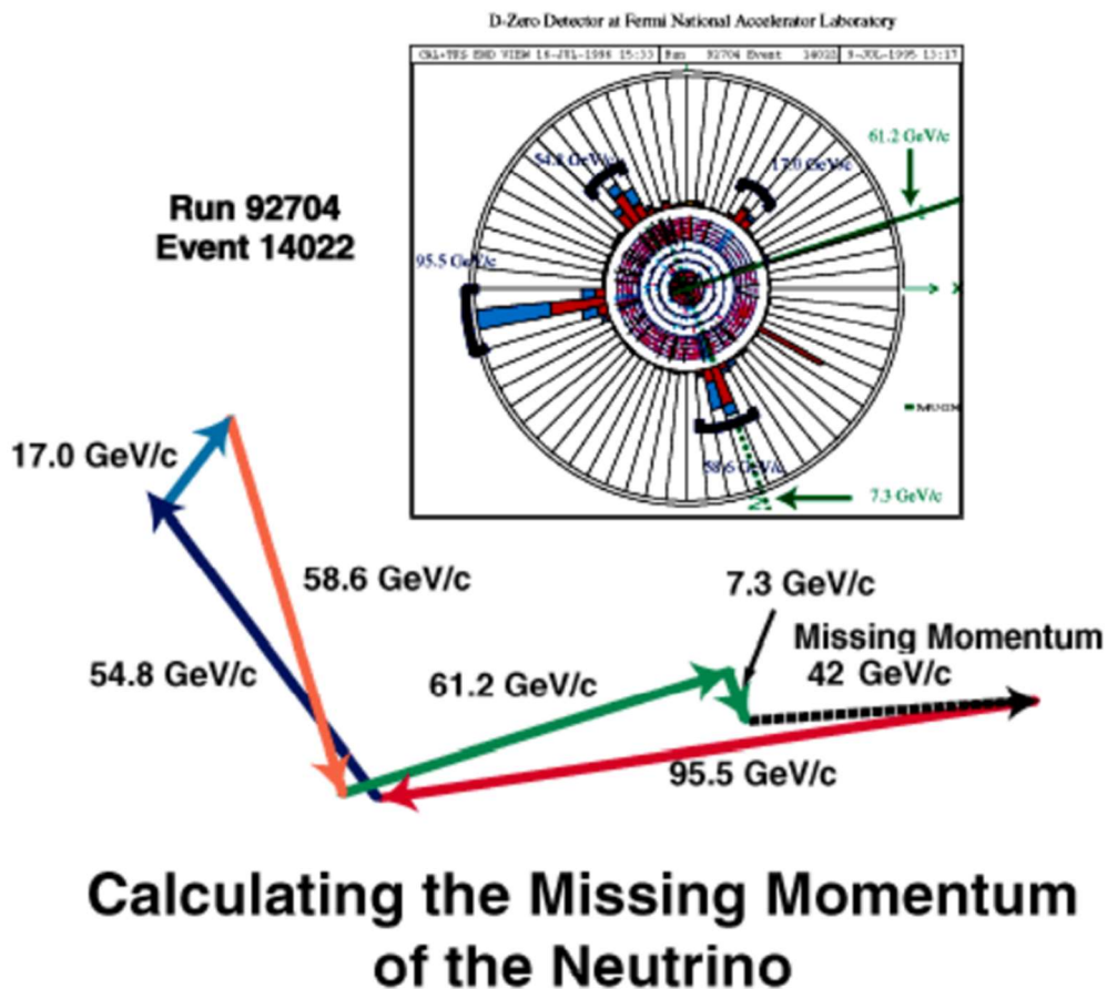
Εικόνα 3 : Απεικόνιση ορμών σωματιδίων
