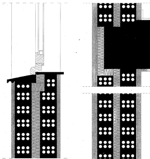
Εικόνα 3: Θερμομόνωση τοιχοποιίας στο διάκενο μεταξύ δύο τοίχων
